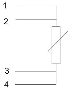
M12-Stecker PT100 1 (braun) 2 (weiss) 3 (blau) 4 (schwarz)
