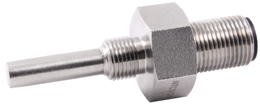
WTR 425OEM-9-G14-50-1A
